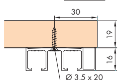
E zum Aufschrauben (nur für 19 mm Türen) for surface mounting with screws (19 mm doors only) à visser en applique (seulement pour portes de 19 mm)
