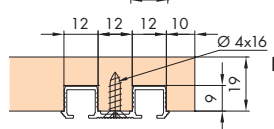
E zum Schrauben for screw fixing à visser
