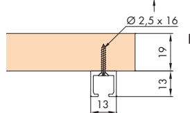
D zum Aufschrauben for surface mounting with screws à visser en applique
