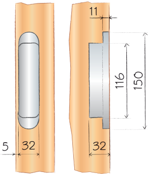
cerniera con e senza meccanismo
