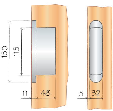
cerniera senza meccanismo
