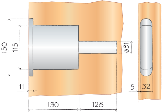
cerniera con meccanismo
