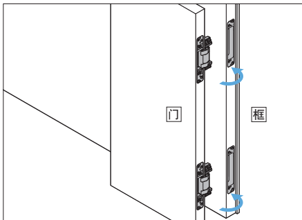
Lapcon门阻尼器LDD-V型 2
